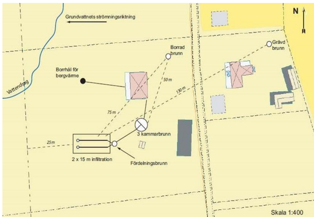
Bild 5 Situationsplan
